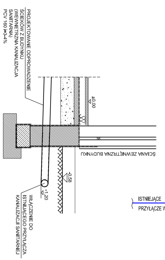
PROFIL PRZYKANALIKA SKALA 1 : 50
